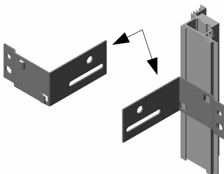
Befestigungswinkel/Staffe di fissaggio/Wall fixing brackets/Étrier de fixation Art. Nr./Item no. 13010a
