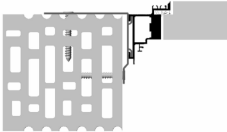
Mod. TCS45/TCS50
